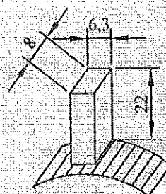
POLOŽAJ ČETKICE
