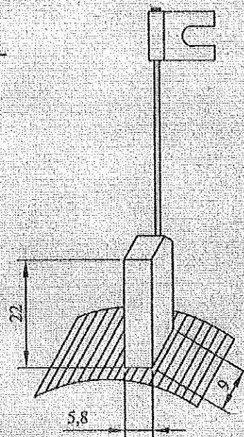
POLOŽAJ ČETKICE
