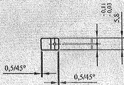
PRESEK B-B
